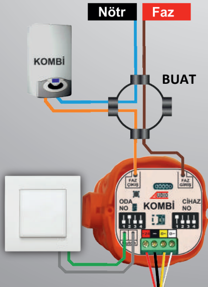
KOMBİ BAĞLANTISI
