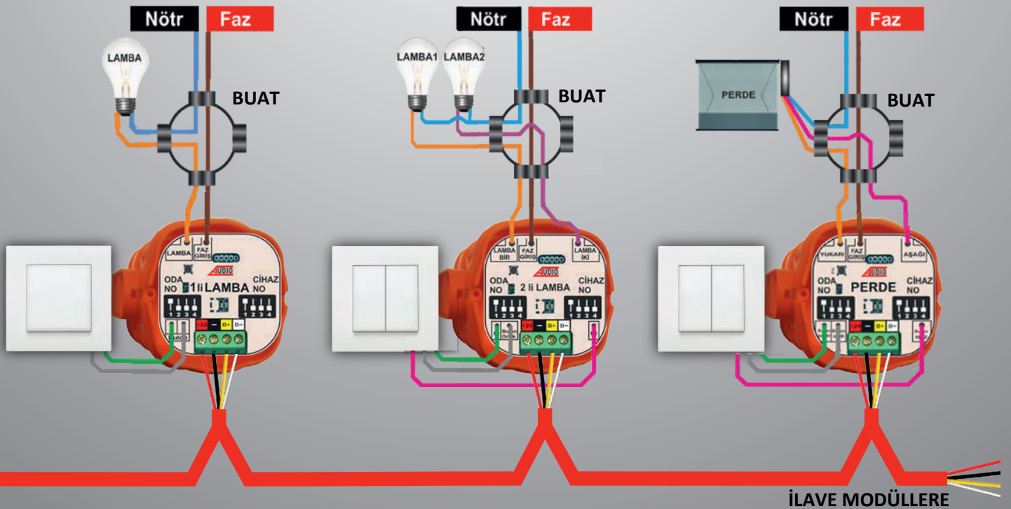
1'li LAMBA BAĞLANTISI
