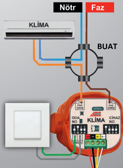
OTOMASYON KABLOSU(OK-4)
